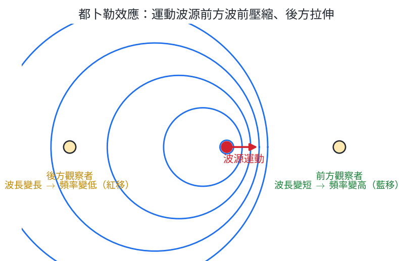
圖 4-6：移動的波源。波源一邊發波一邊前進，使前方的波前一個個擠近（波長短、頻率高，藍移），後方的波前被拉開（波長長、頻率低，紅移）。
