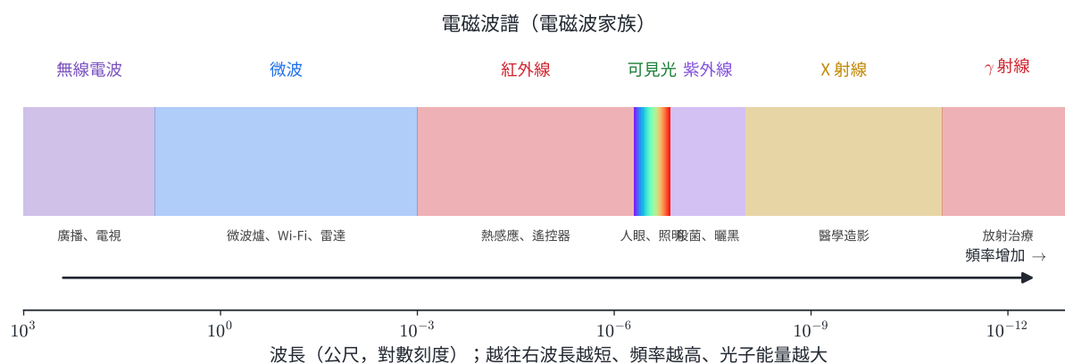
圖 4-5：電磁波譜（橫軸為波長，對數刻度）。由左到右波長漸短、頻率漸高、光子能量漸大：無線電波 → 微波 → 紅外線 → 可見光 → 紫外線 → X 射線 → \gamma 射線。可見光只占其中極窄的一段。
